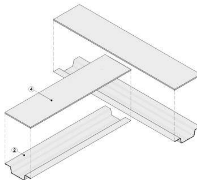
Vista isométrica
