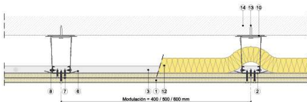
Sección vertical
