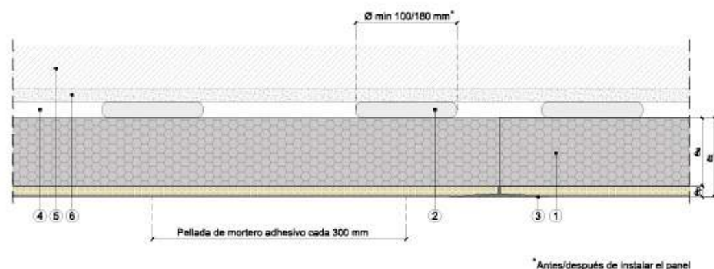
Sección horizontal
