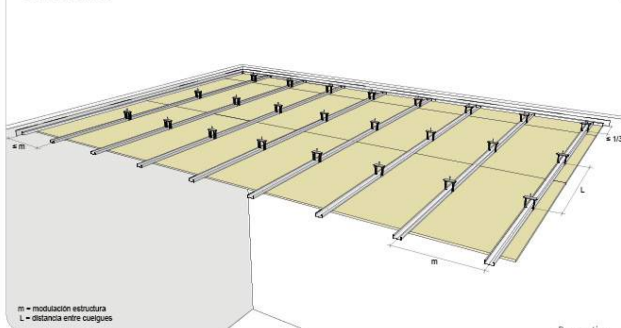
Perspectiva
