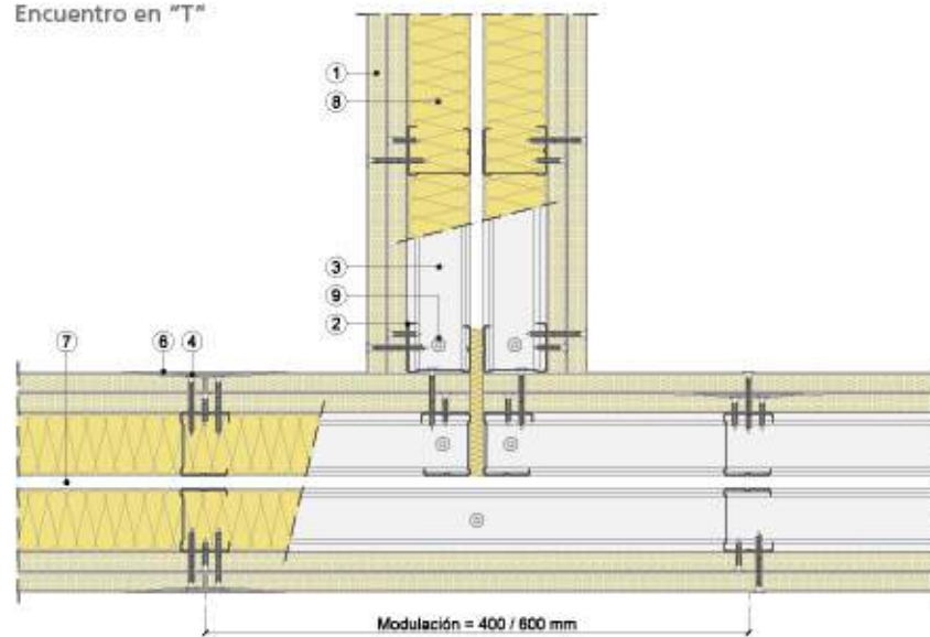
Encuentro en "T"
