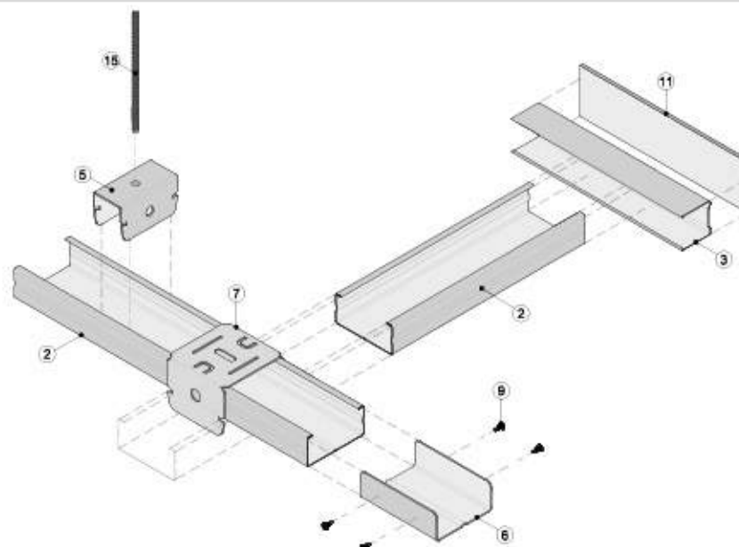
Vista isométrica
