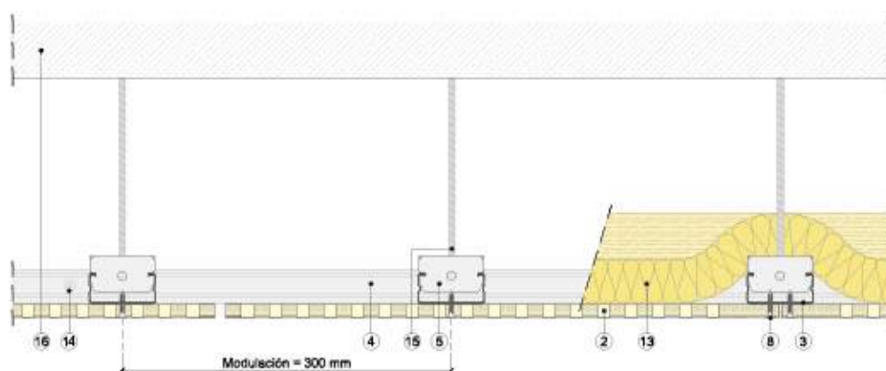
Sección vertical
