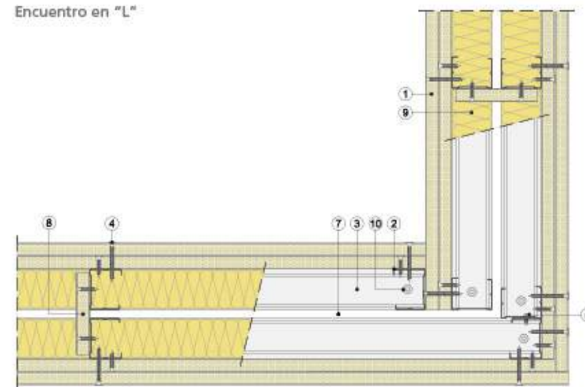
Encuentro en "L"
