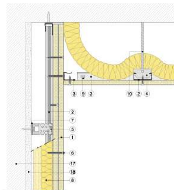
Sección vertical
