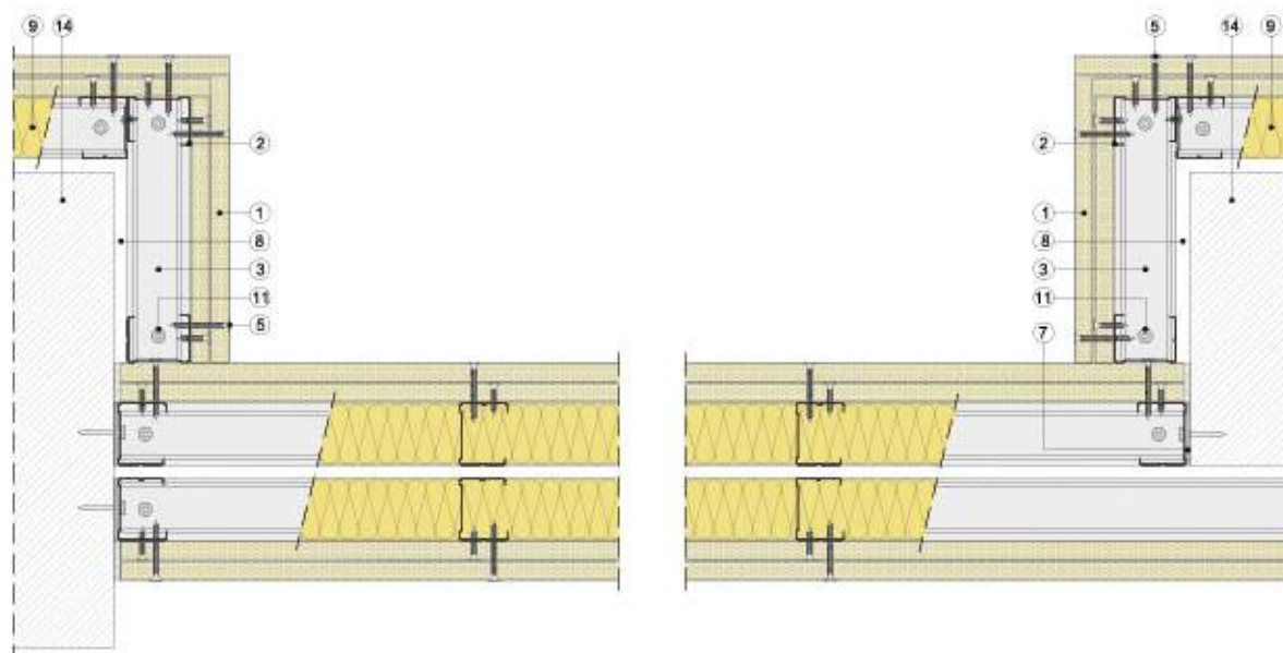
Sección horizontal
