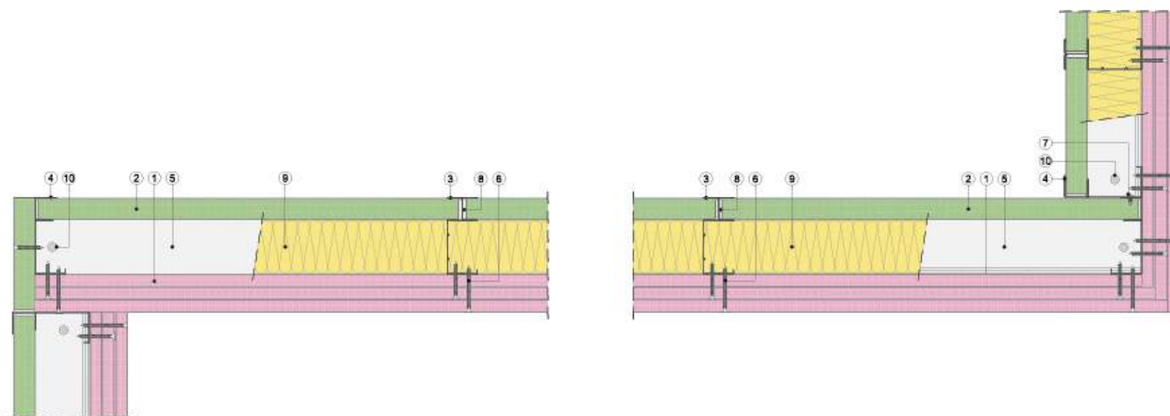
Sección horizontal
