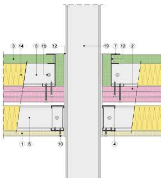
Sección horizontal
