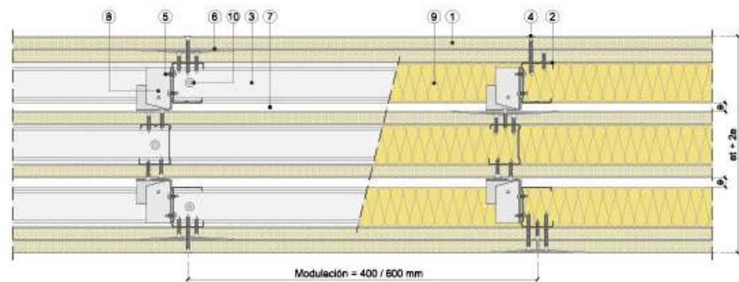
Sección horizontal
