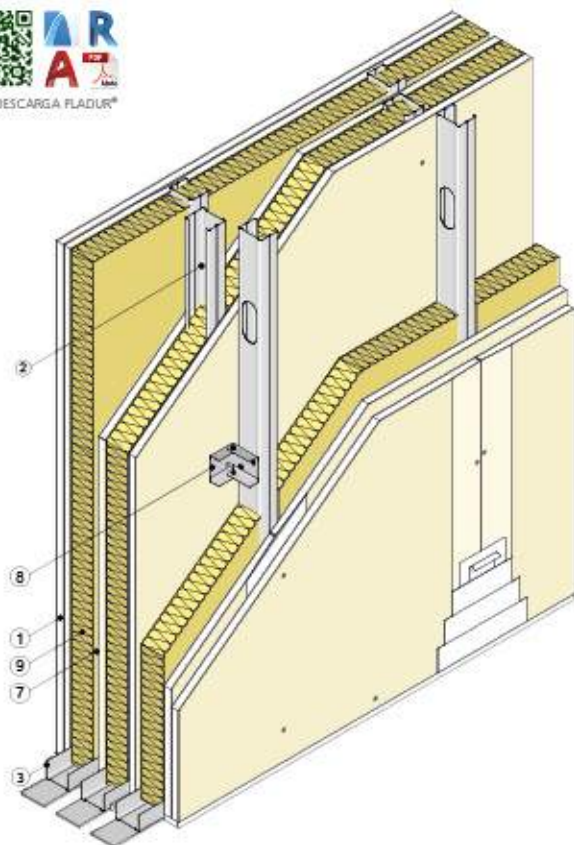
Vista isométrica
