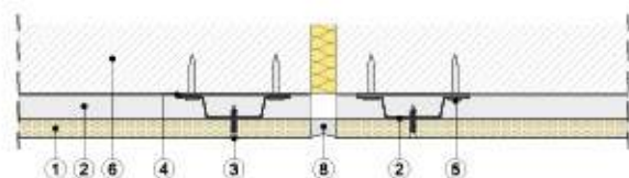
Sección horizontal
