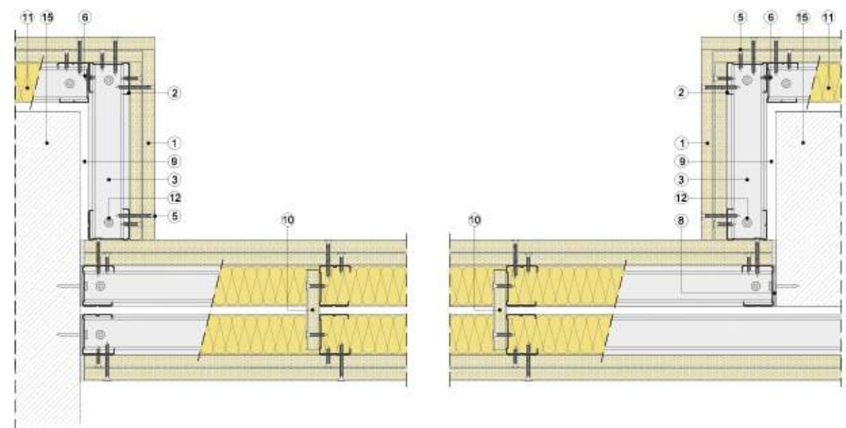
Sección horizontal
