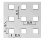
Diseño de perforado
