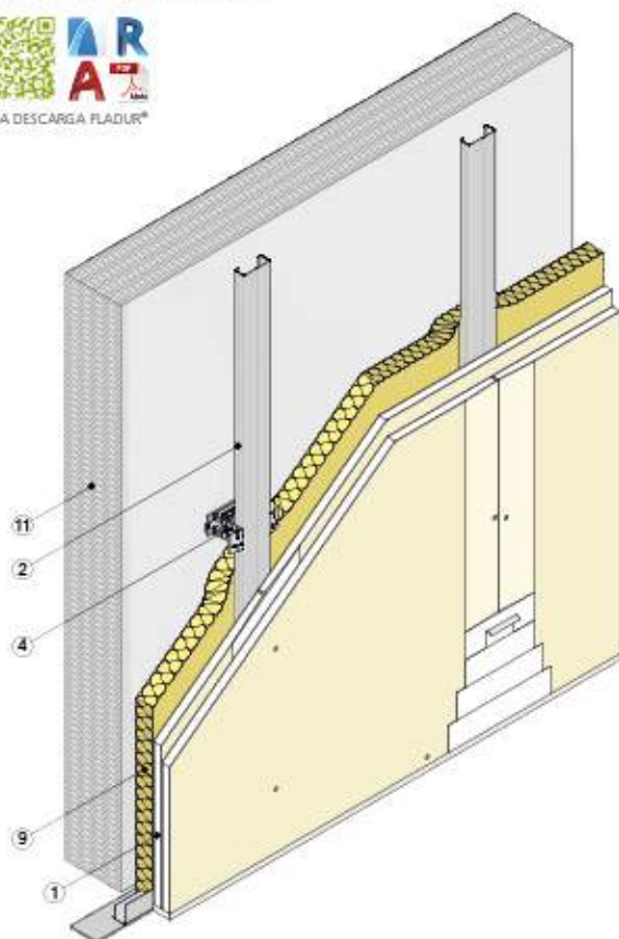
Vista isométrica
