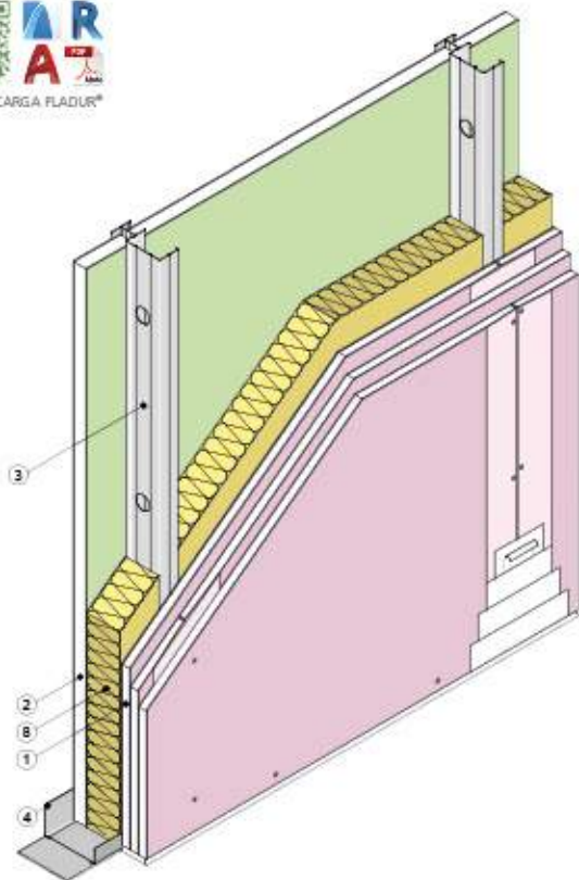
Vista isométrica
