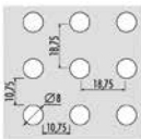
Diseño de perforado
