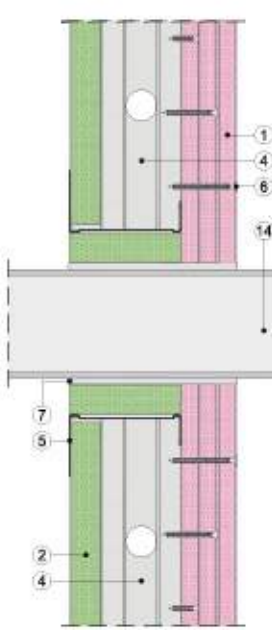
Sección vertical
