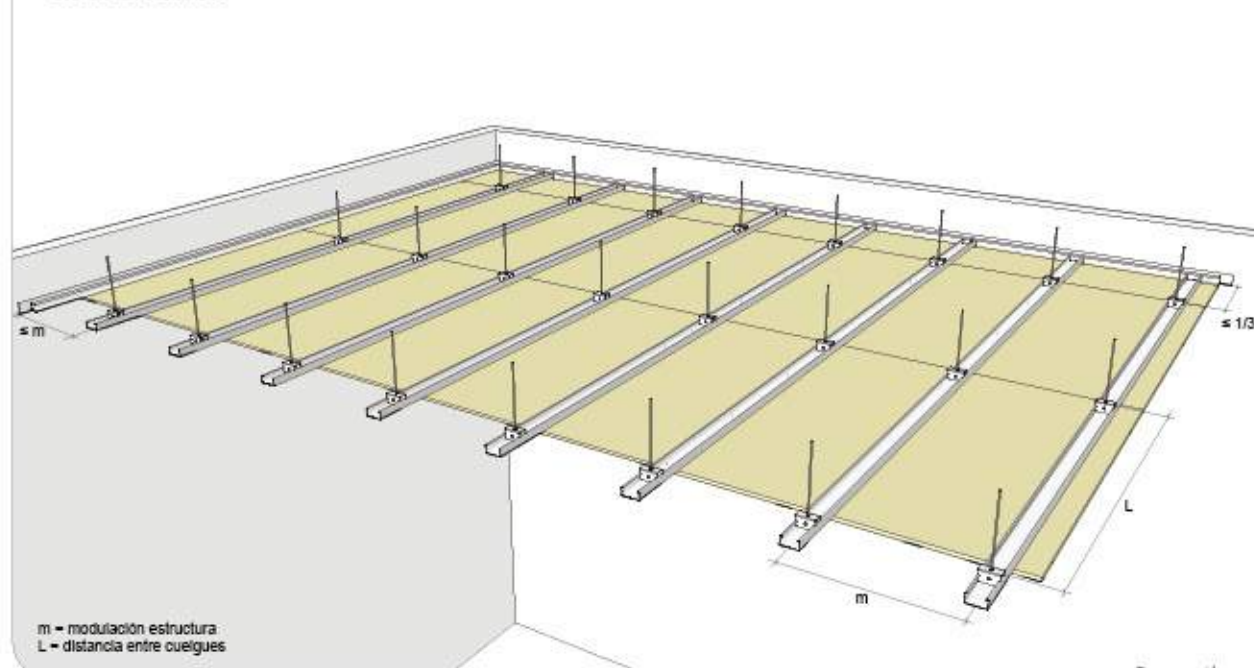
Perspectiva
