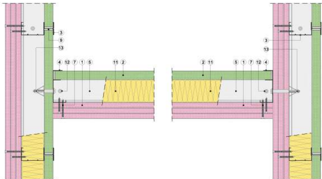
Sección horizontal
