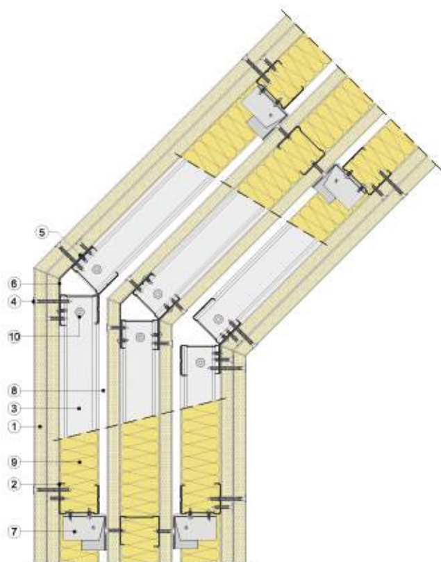
Sección horizontal
