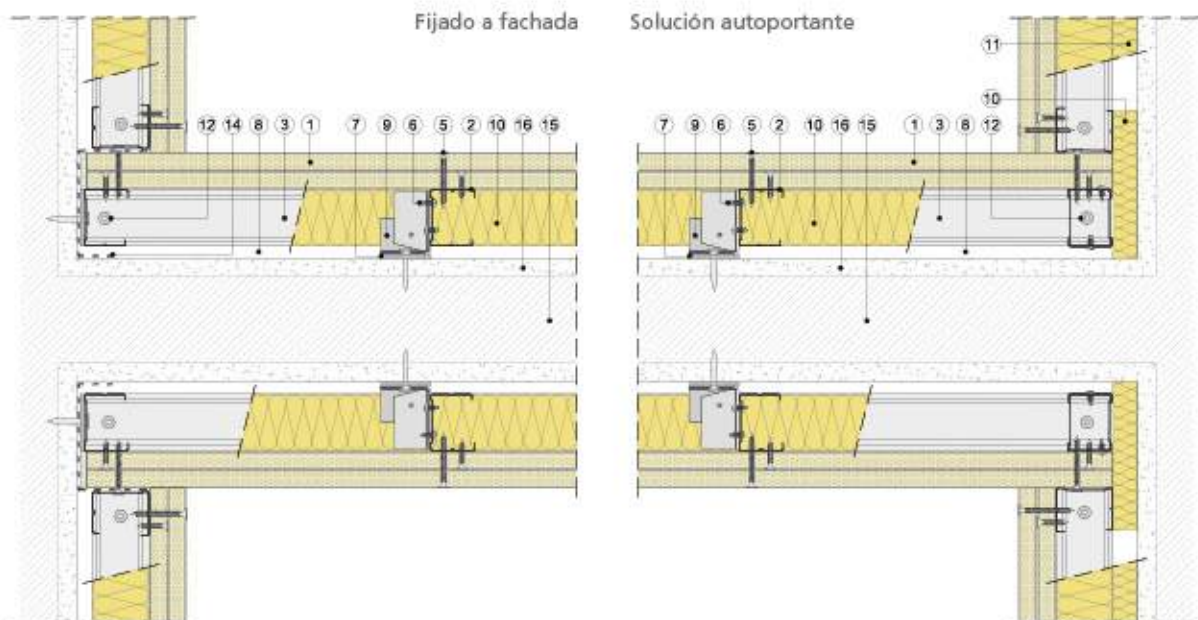
Sección horizontal
