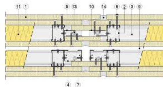
Sección horizontal
