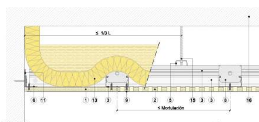
Sección transversal
