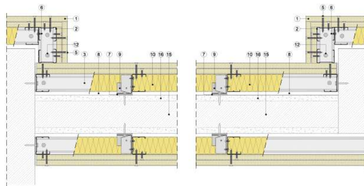
Sección horizontal
