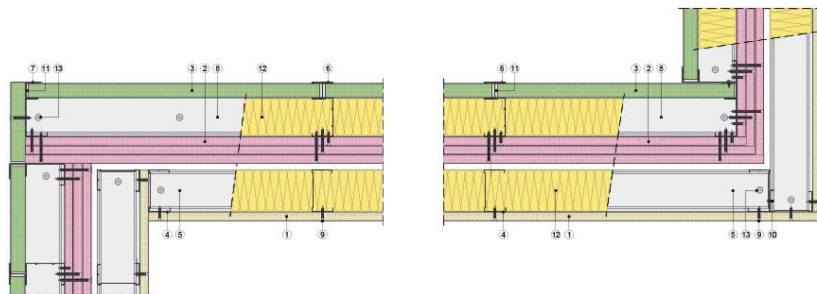
Sección horizontal
