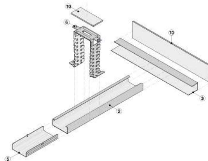
Vista isométrica
