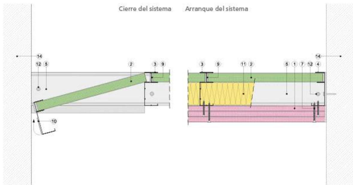
Sección horizontal
