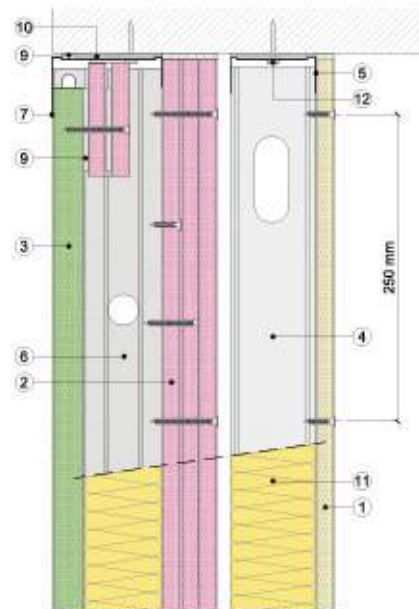
Sección vertical
