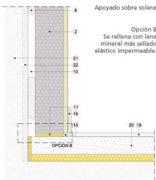
Sección vertical
