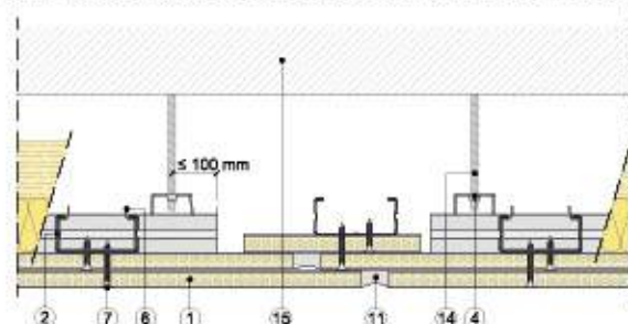
Sección vertical
