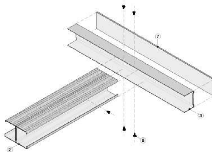
Vista isométrica
