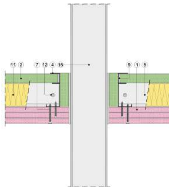
Sección horizontal
