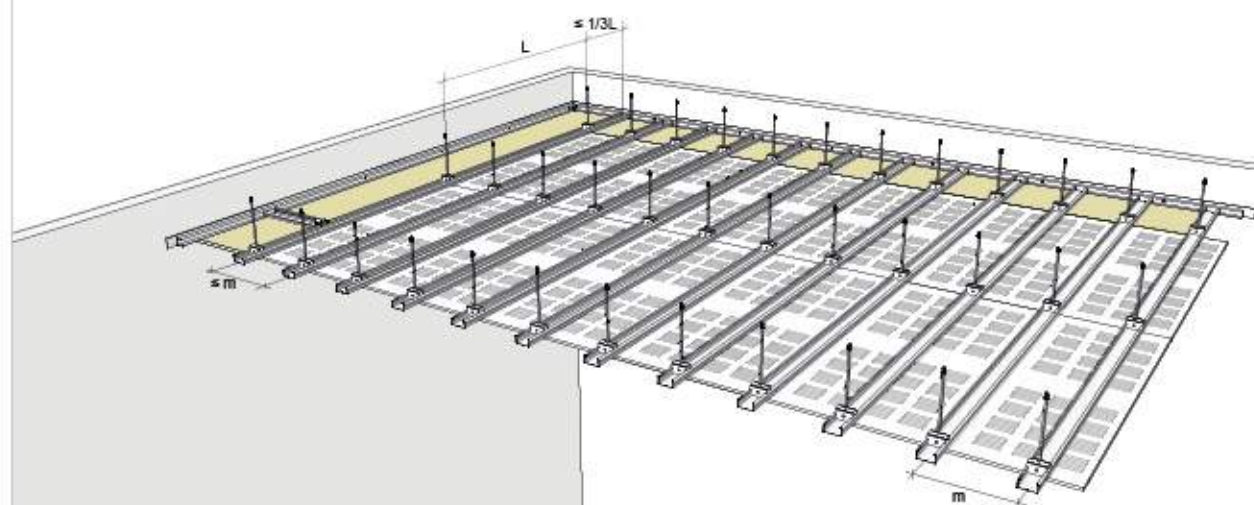
Perspectiva
