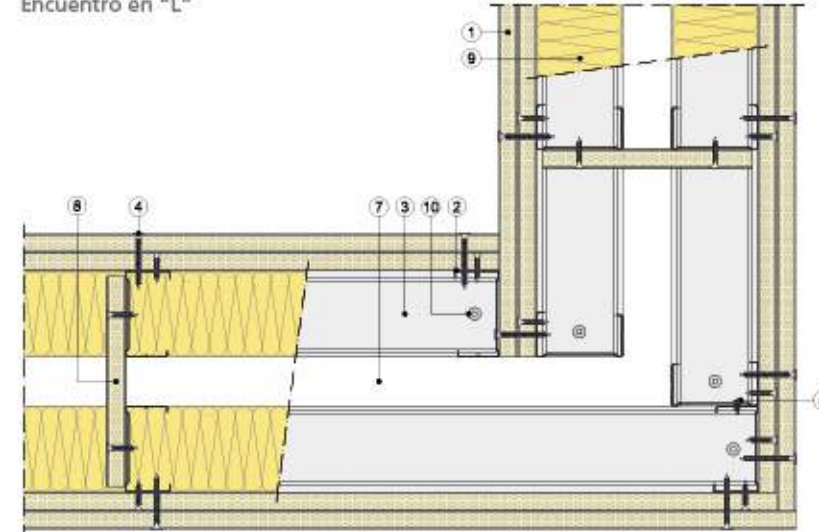
Encuentro en "L"
