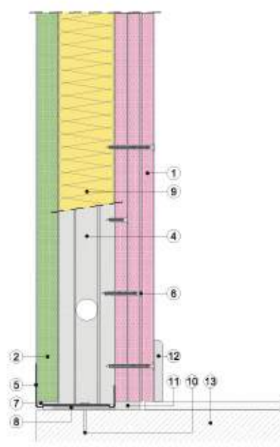
Sección vertical
