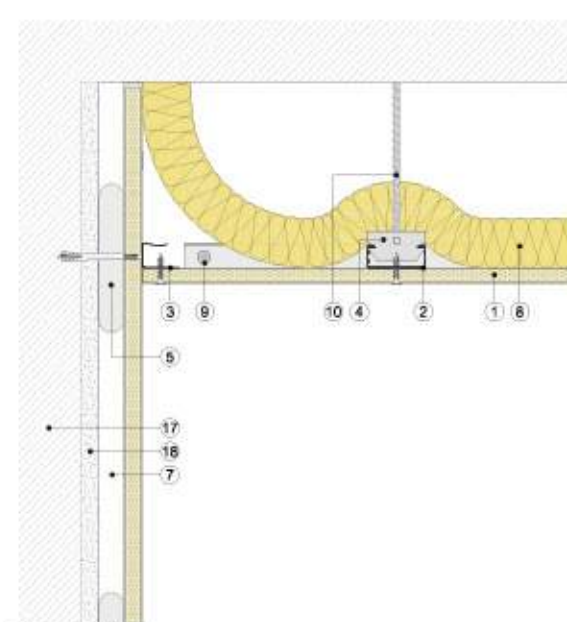
Sección vertical
