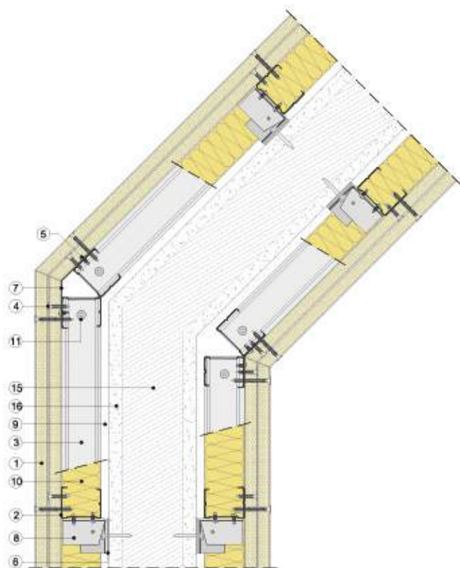
Sección horizontal
