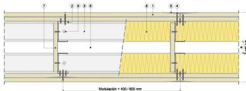
Sección horizontal
