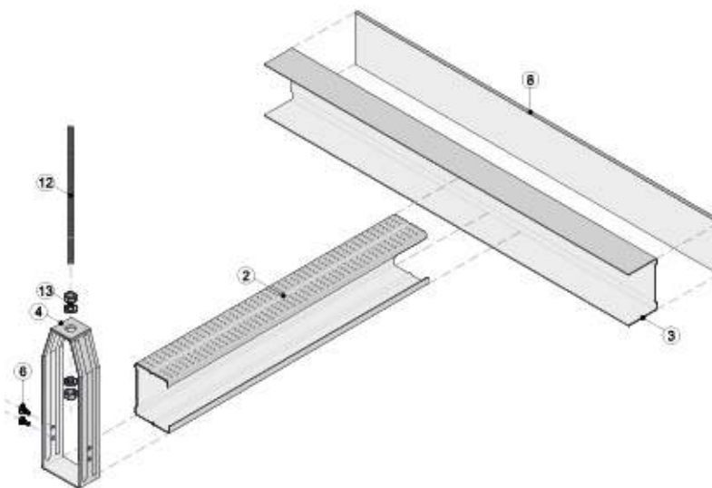
Vista isométrica
