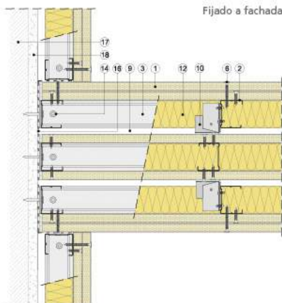
Fijado a fachada
