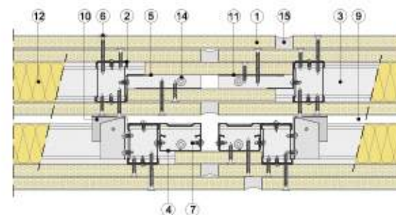
Sección horizontal
