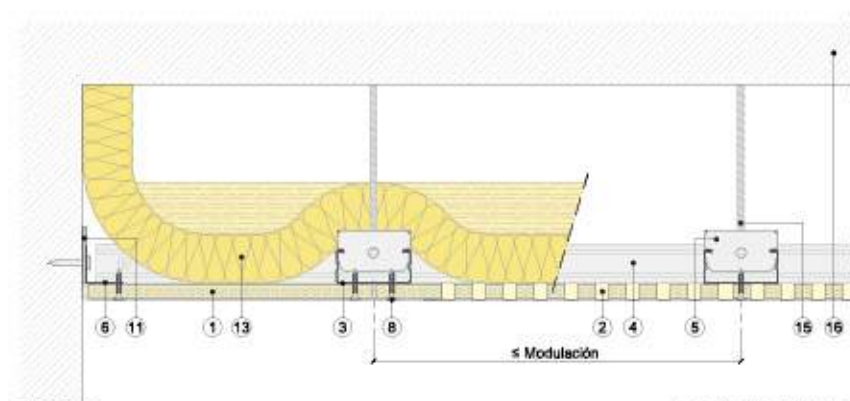
Sección transversal
