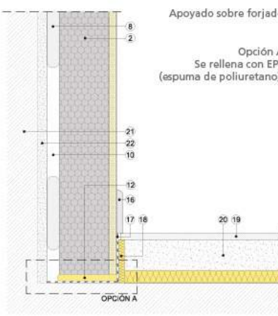
Sección vertical
