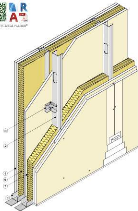
Vista isométrica
