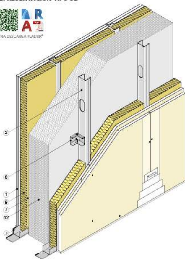
Vista isométrica
