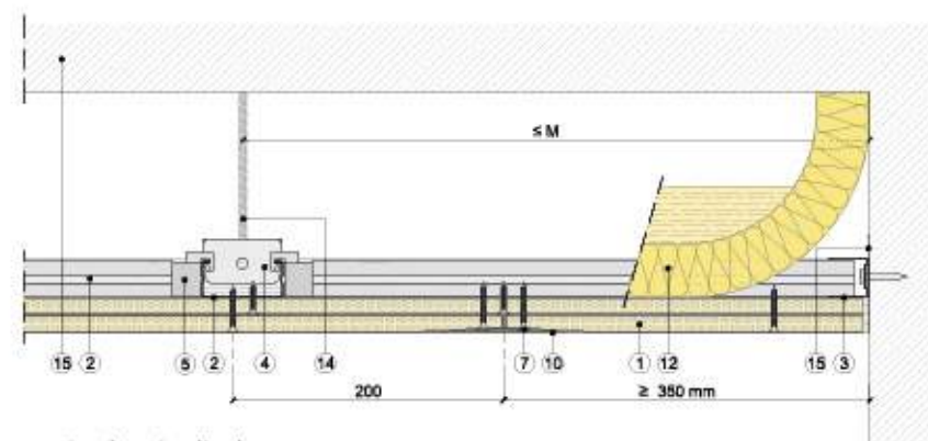
Sección longitudinal
