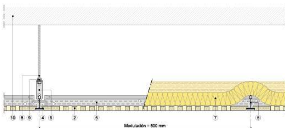
Sección vertical
