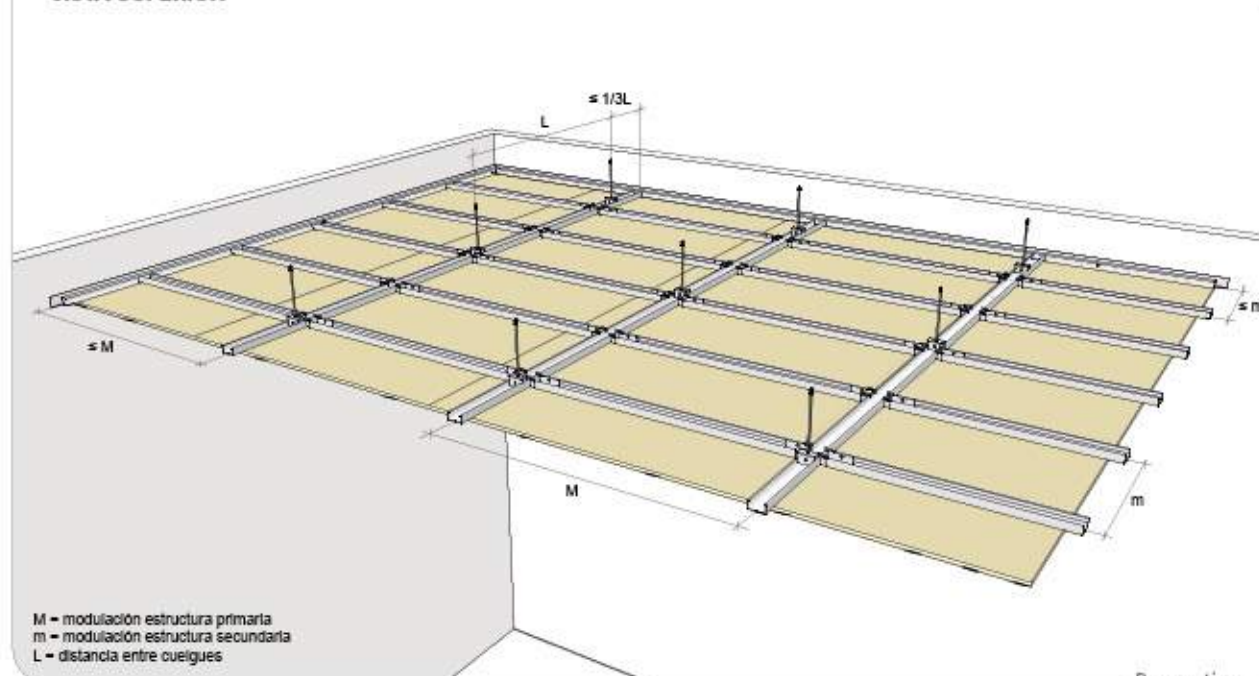
Perspectiva
