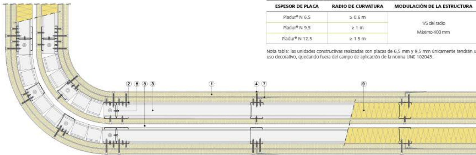
Sección horizontal
