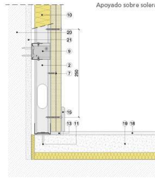
Sección vertical
