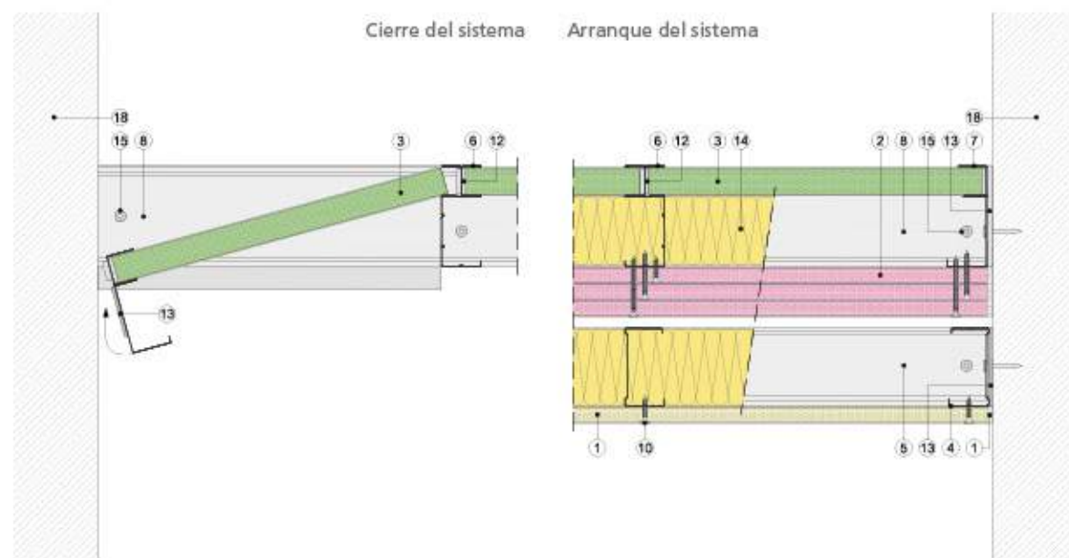
Sección horizontal
