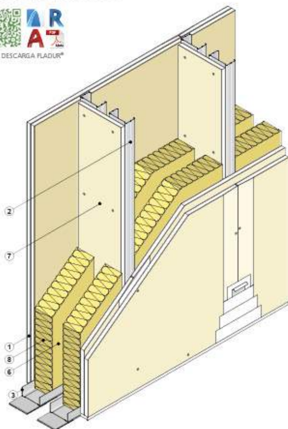
Vista isométrica
