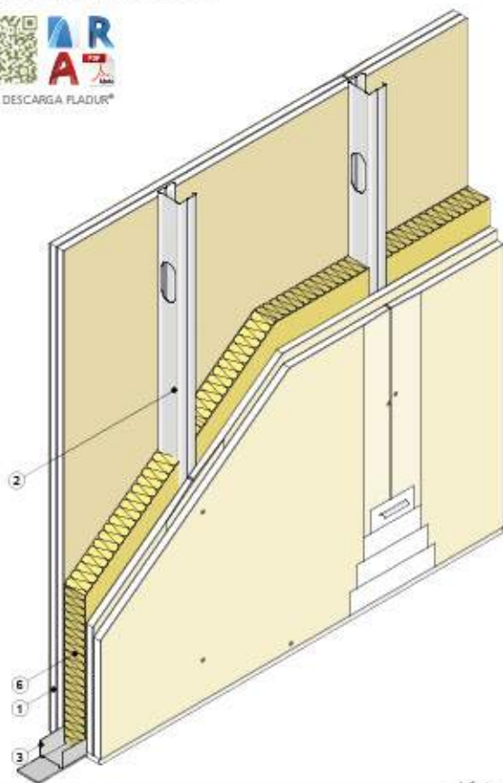
Vista isométrica
