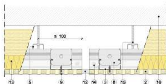
Sección vertical
