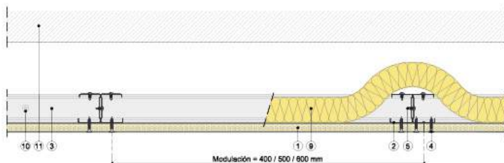
Sección vertical
