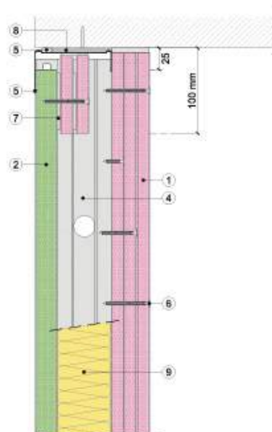
Sección vertical
