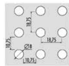
Diseño de perforado
