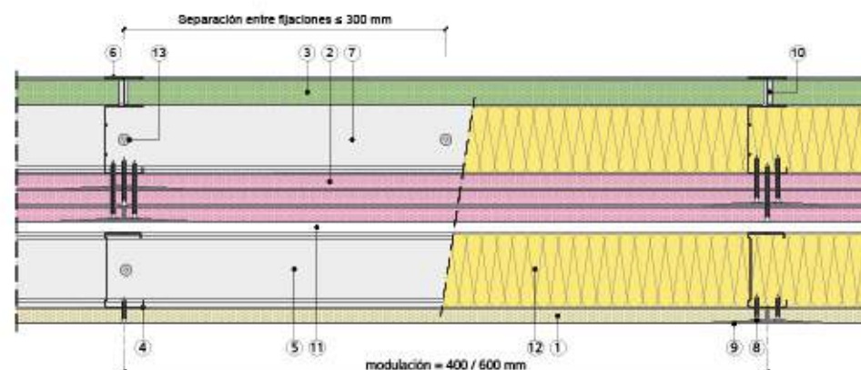
Sección horizontal
