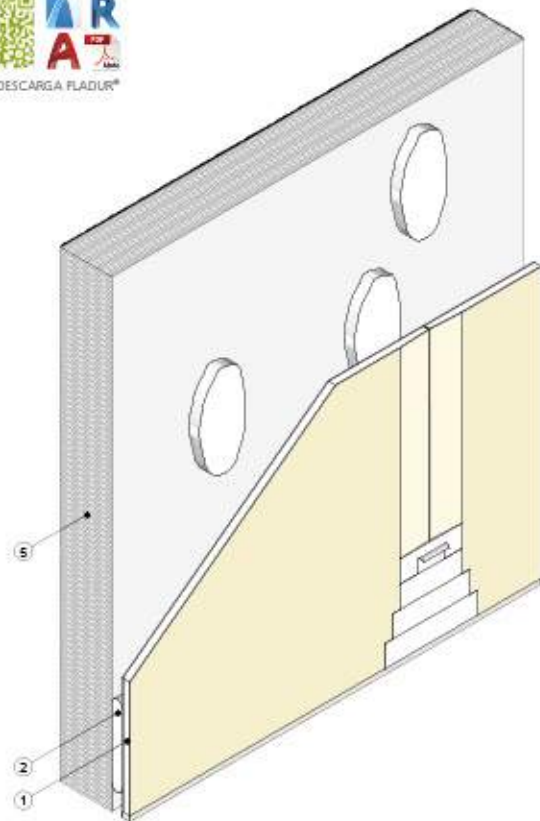
Vista isométrica
