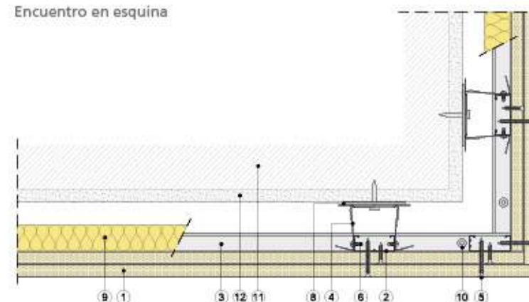
Encuentro en esquina
