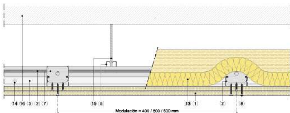
Sección vertical
