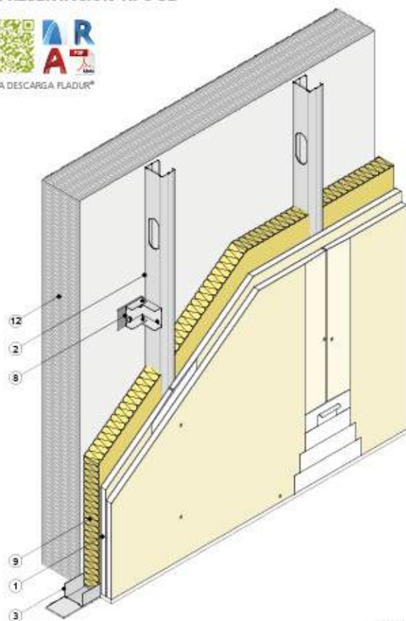
Vista isométrica
