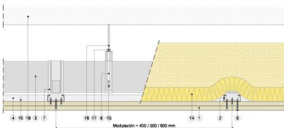
Sección vertical
