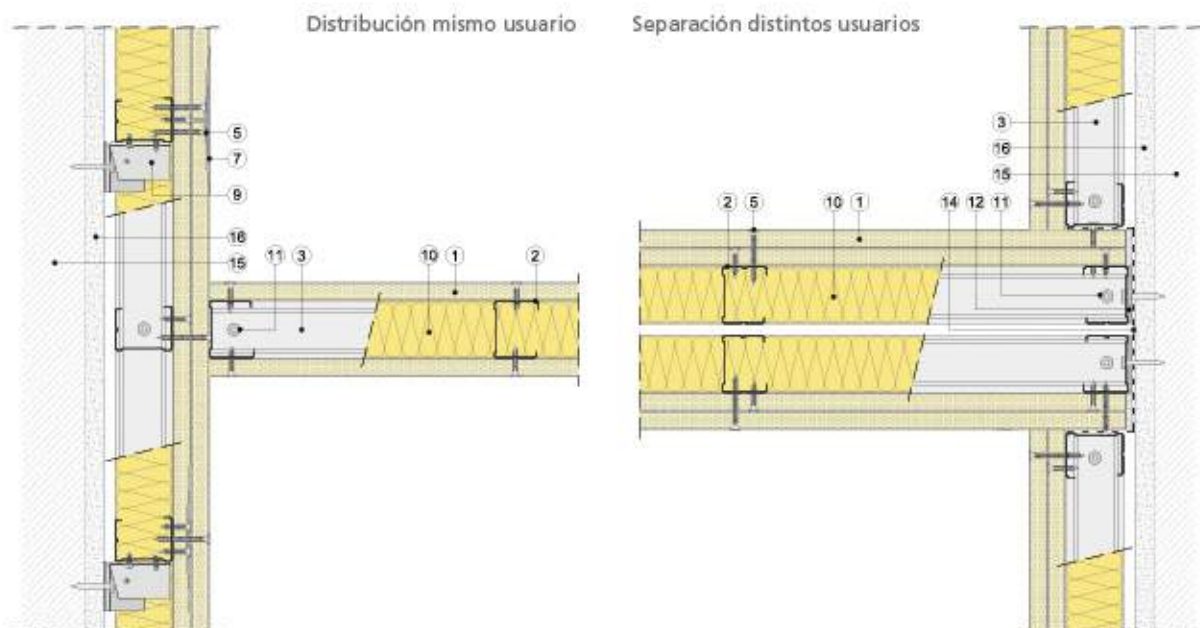
Sección horizontal
