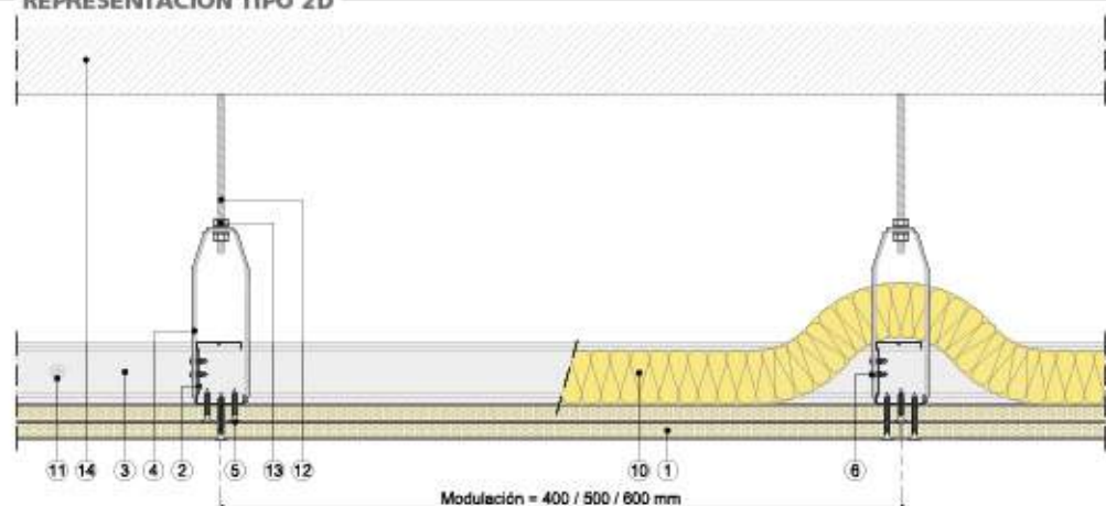
Sección vertical
