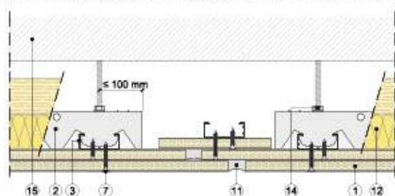
Sección vertical
