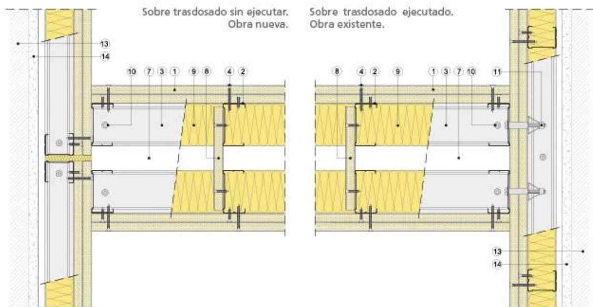
Sección horizontal
