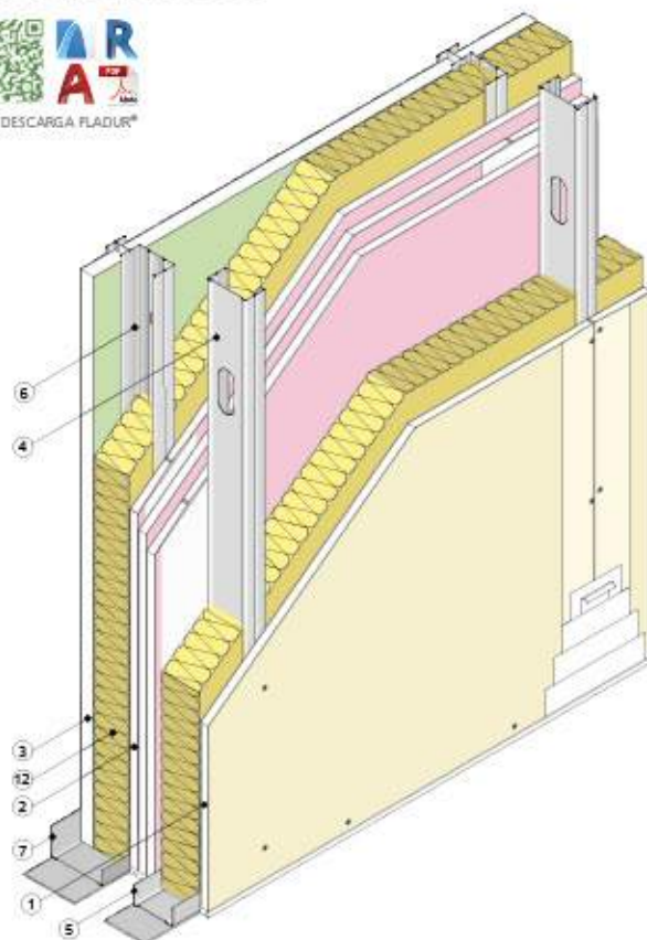
Vista isométrica
