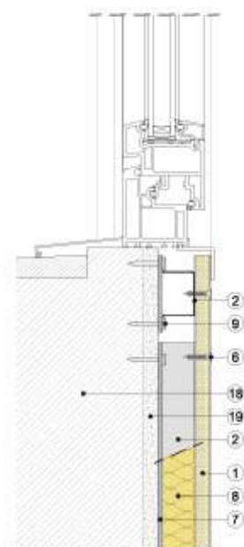
Encuentro con antepecho
