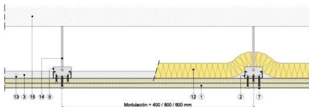
Sección vertical
