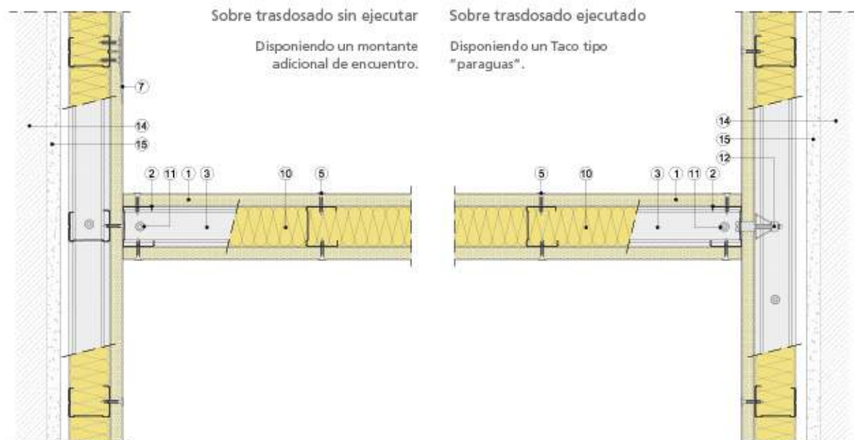
Sección horizontal
