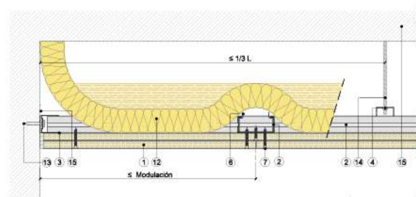
Sección transversal
