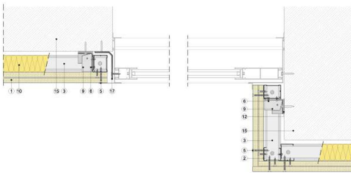
Sección horizontal
