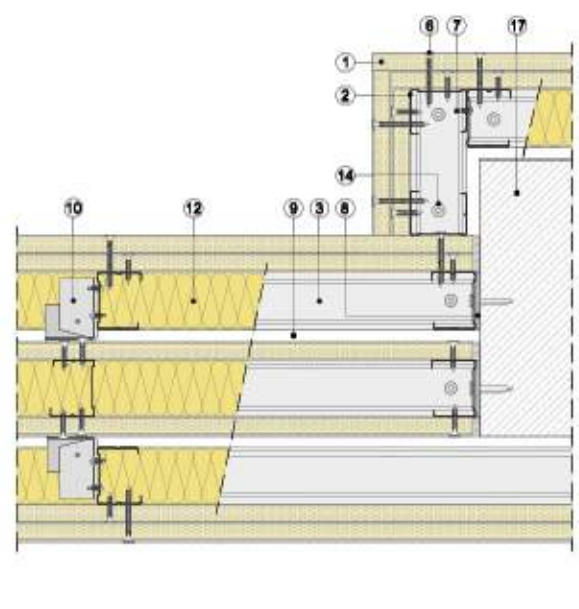
Sección horizontal
