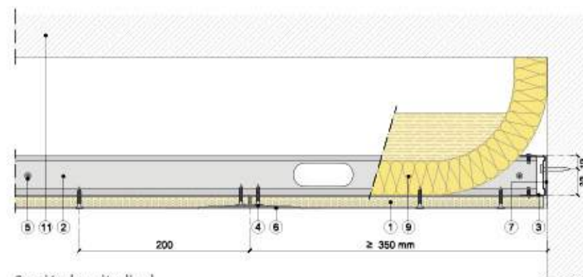
Sección longitudinal
