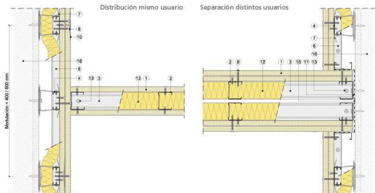
Sección horizontal
