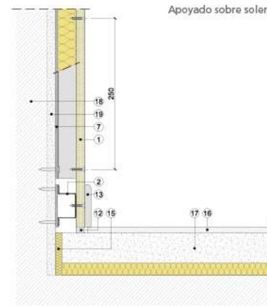
Sección vertical
