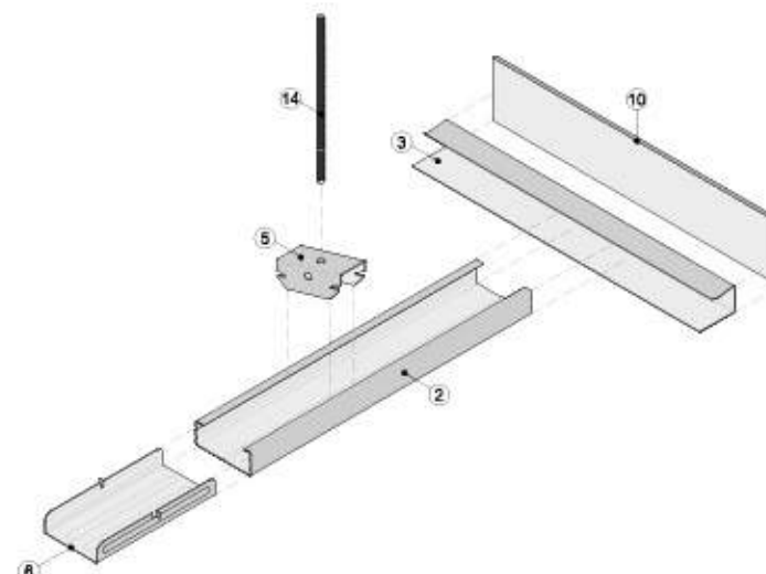
Vista isométrica
