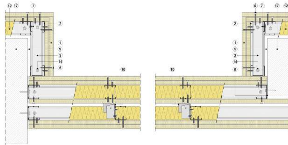
Sección horizontal
