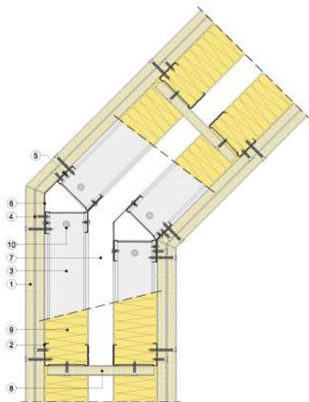
Sección horizontal
