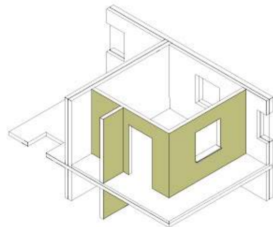
ESTRUCTURA SIMPLE - TABIQUE PLADUR® SENCILLO (P. 240)
