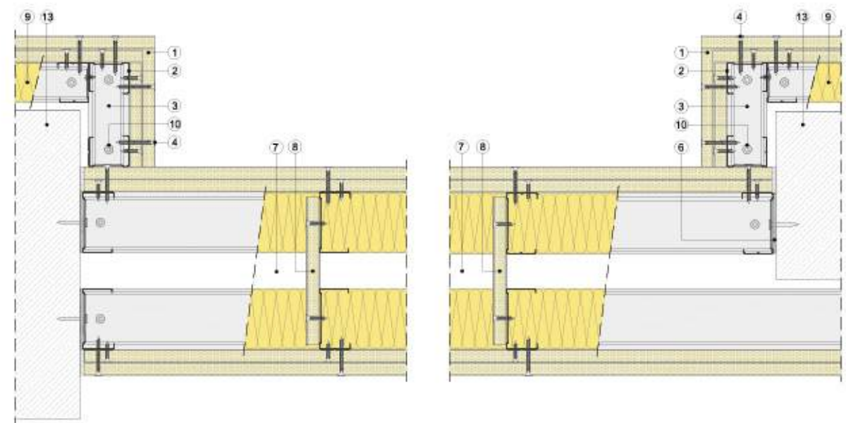
Sección horizontal
