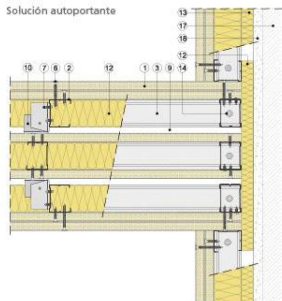
Sección horizontal
