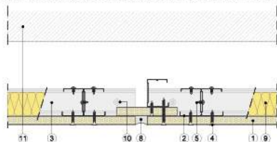
Sección vertical
