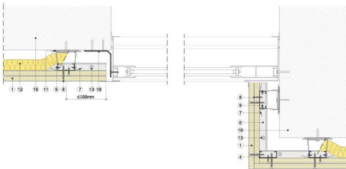
Sección horizontal
