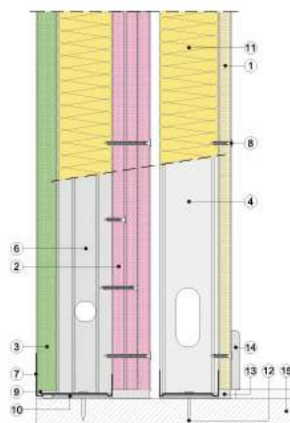
Sección vertical
