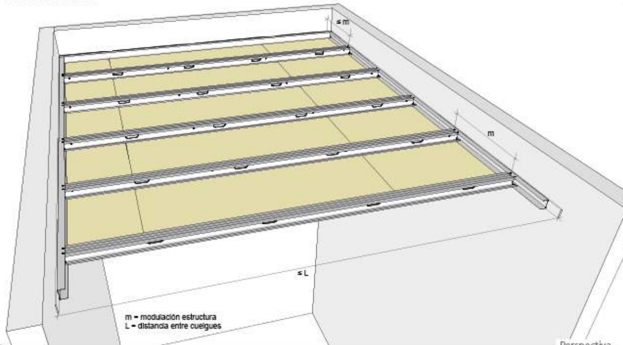
Perspectiva
