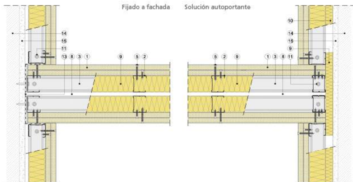
Sección horizontal
