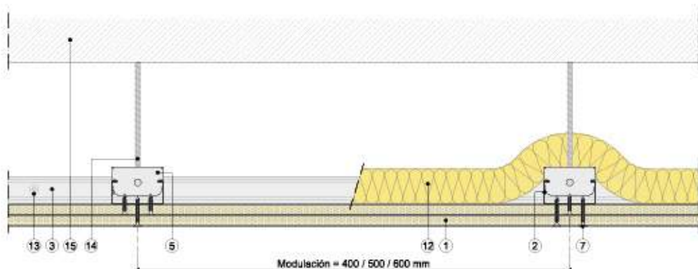
Sección vertical
