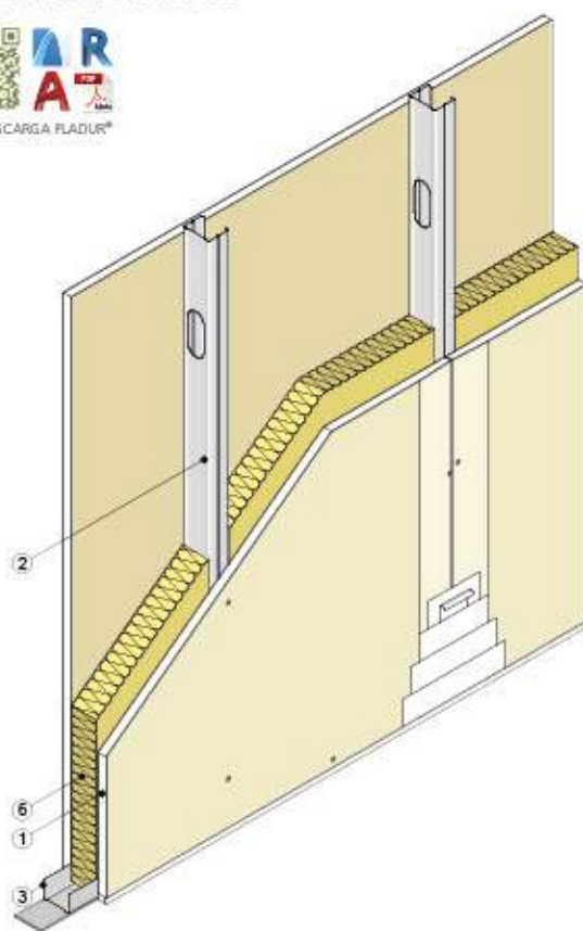
Vista isométrica
