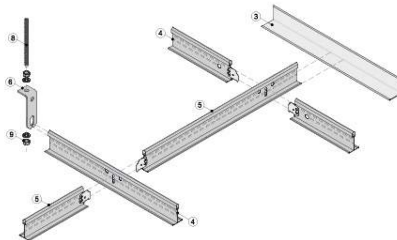
Vista isométrica
