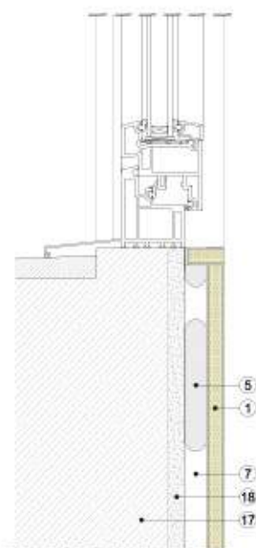
Encuentro con antepecho
