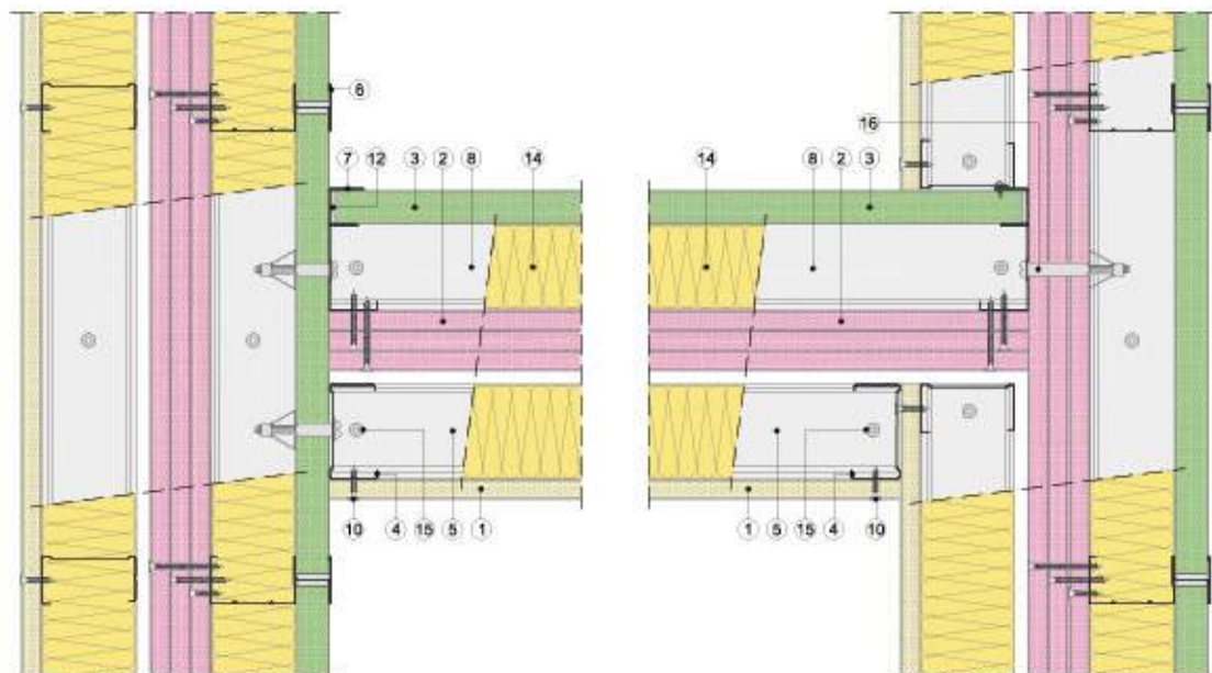
Sección horizontal
