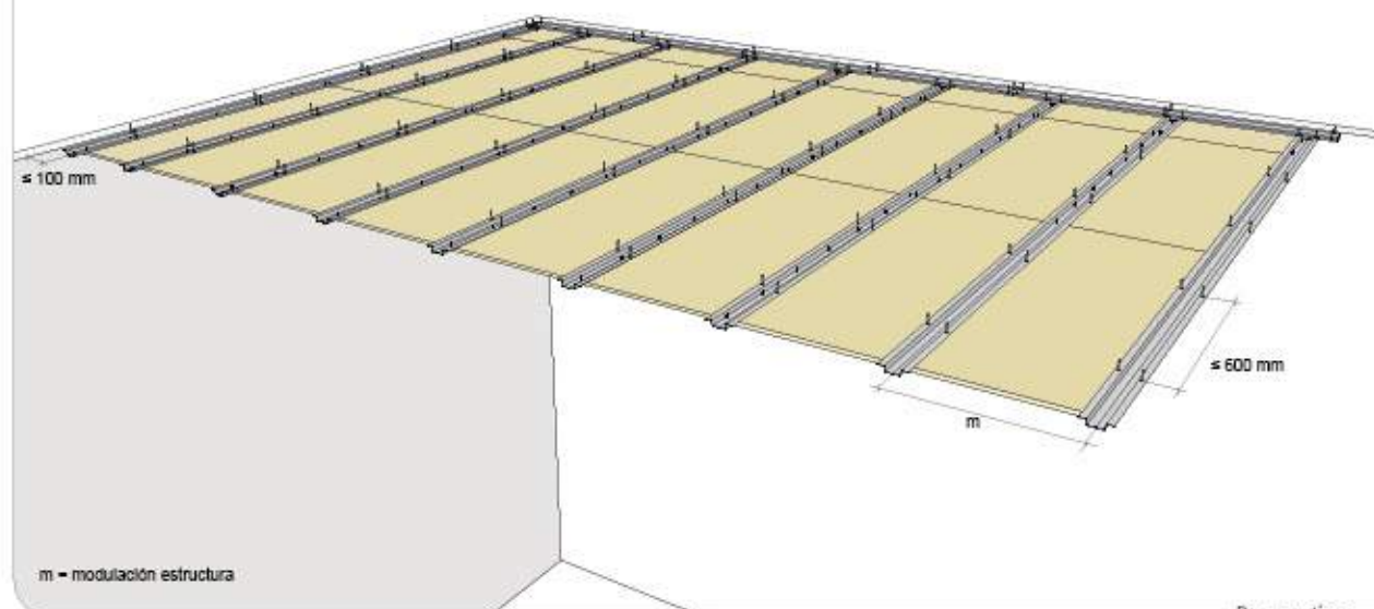
Perspectiva
