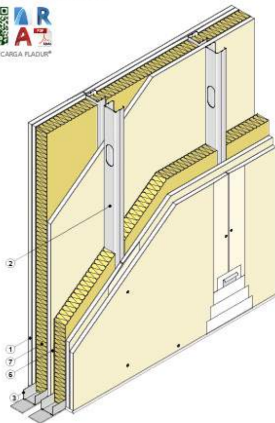
Vista isométrica
