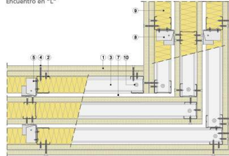
Encuentro en "L"
