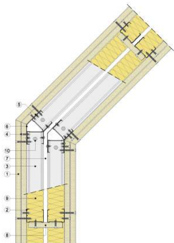
Sección horizontal
