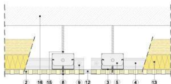
Sección vertical
