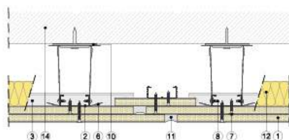
Sección vertical
